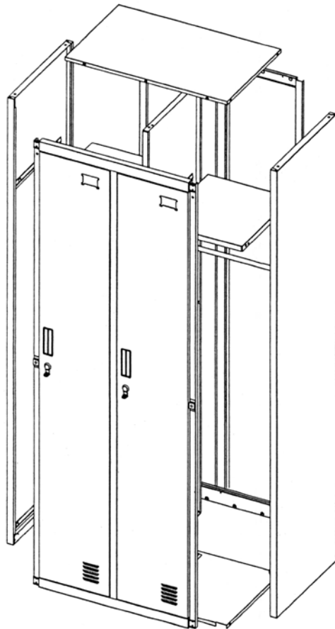
Right Side:1Pc
